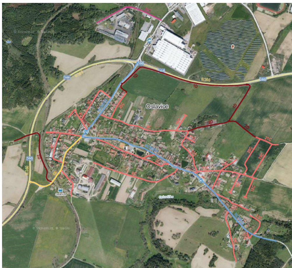
Pasportizované komunikace v obci vč. označení a klasifikace
